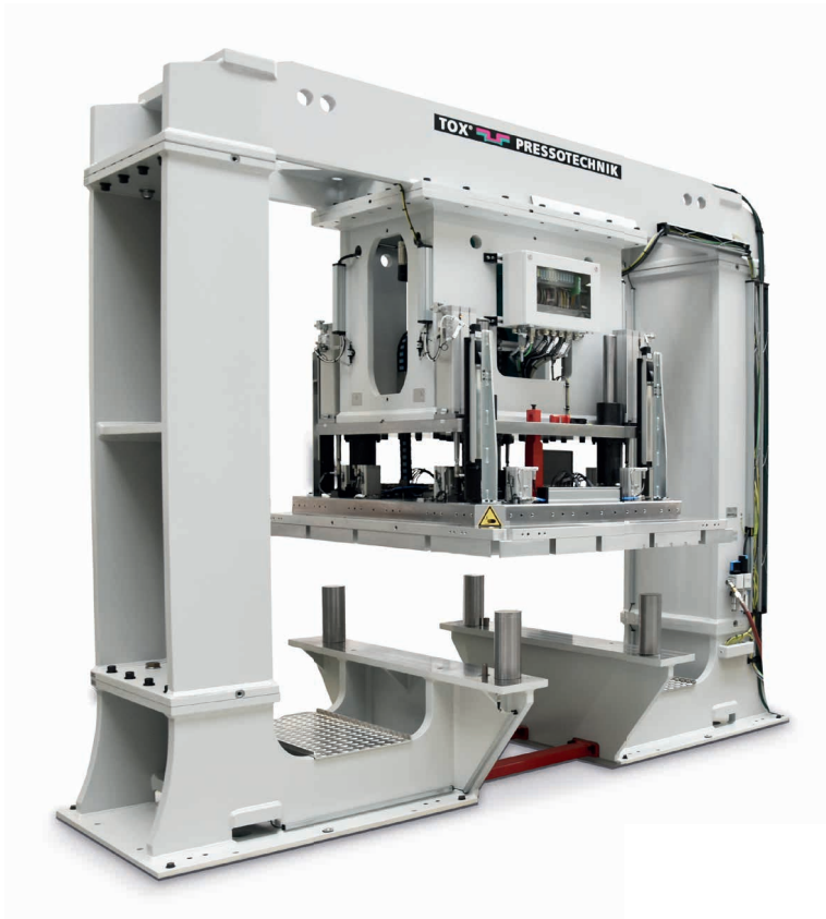
TOX®-Pressensystem Baureihe MAG mit elektromechanischem Antrieb TOX®-ElectricDrive
